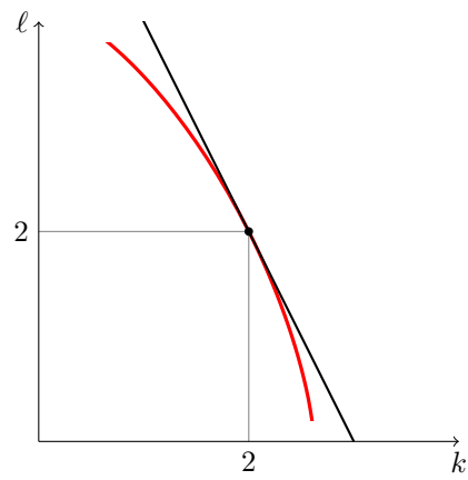
Figure 4: CET Choice
